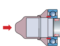
Použití vhodného montážního nářadí zabraňuje poškození oběžných drah.
