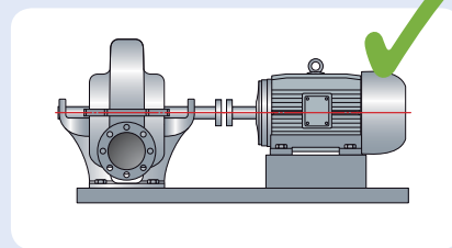
Správné ustavení
