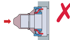
Působení montážní síly na nesprávný kroužek ložiska může způsobit poškození oběžných drah.
