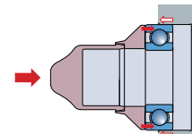
Použití vhodného montážního nářadí zabraňuje poškození oběžných drah.
