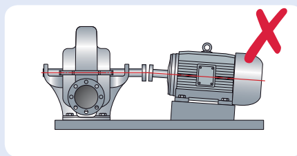
Úhlová nesouosost
